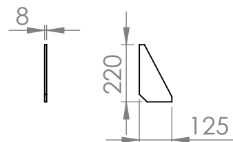
détail de gousset
